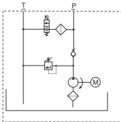
Hyd. Schematic
